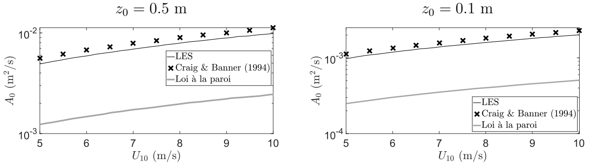
FIGURE 1.29 – Diffusivité turbulente, A_0 , dans la zone de déferlement des vagues ( z \sim 0 ), en fonction de la vitesse du vent, U_{10} , mesurée à 10 m au-dessus de la surface de l'eau. Le trait plein noir correspond aux données LES obtenues par Kukulka & Brunner (2015), celui gris correspond aux valeurs déduites par le modèle classique de la loi à la paroi et les croix sont les valeurs obtenues par le modèle eq. (1.21). Figure adaptée de Kukulka & Brunner (2015) pour deux hauteurs de rugosité z_0 .
