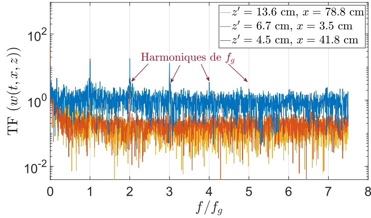
FIGURE 2.34 – (a) Spectre temporel du champ instantané de la vitesse verticale, w(t, x, z) , à trois positions distinctes. La fréquence est normalisée par la fréquence de la grille, f_g .
