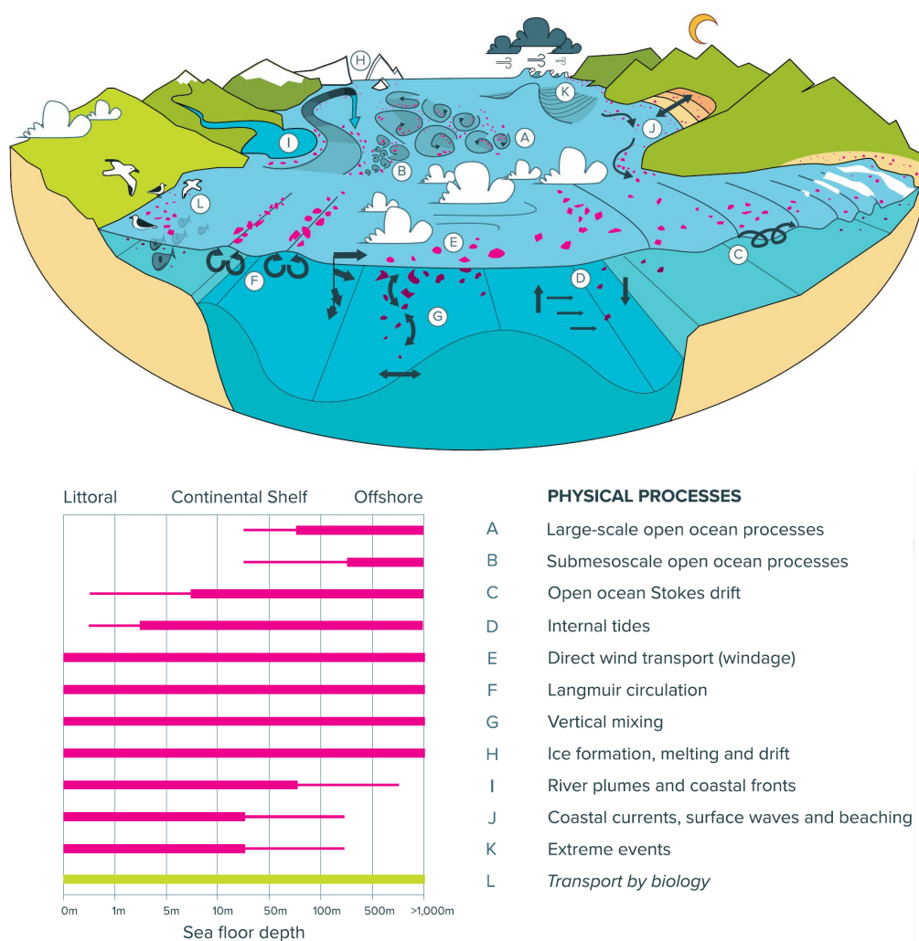
FIGURE 1.26 – Représentation schématique des processus océaniques générant de la turbulence (haut de la figure). La Table (bas de la figure) indique l'importance relative de chaque processus sur le transport des plastiques en fonction des régions (littoral, côtier ou haute mer). L'épaisseur des traits indique le degré d'importance (trait épais = importance élevée et trait fin = importance moindre). Le transport par la voie biologique n'étant pas un processus physique, il a été représenté en vert. Figure tirée de Van Sebille et al. (2020).
