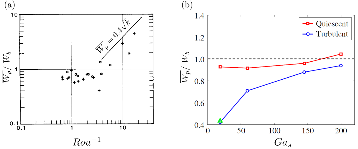
FIGURE 1.18 – (a) Vitesse moyenne de remontée d’une particule dans un écoulement turbulent, W_p , normalisée par la vitesse de Stokes, W_b , en fonction de l’inverse du nombre de Rouse, Rou . Figure adaptée de Nielsen (1993). (b) Rapport de W_p/W_b en fonction du nombre de Galilée, Ga . Figure adaptée de Fornari et al. (2016b).
