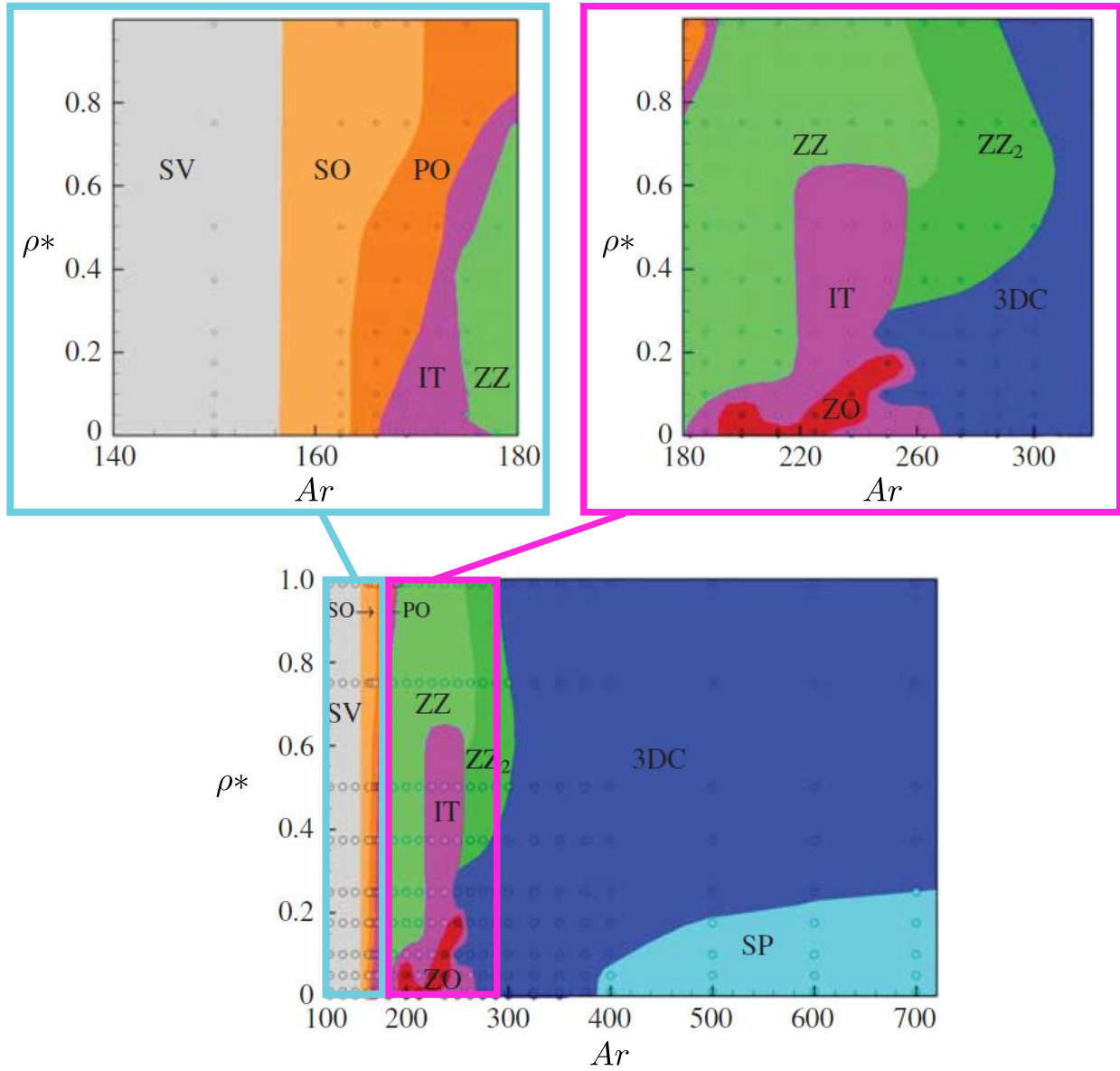
Figure S1 – Carte des transition de sillage d'une sphère remontant dans un fluide. SV : Steady Vertical, SO : Steady Oblique, PO : Periodic Oblique, IT : Intermitent, ZZ : Zig-Zag, ZZ 2 : small amplitdute Zig-Zag, ZO : Zig-Zag Oblique, 3DC : Tree Dimensional Chaotic, SP : Spiraling. Figure adaptée de Auguste & Magnaudet (2018).
