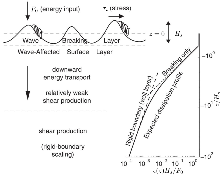
FIGURE 1.28 – Représentation schématique de la couche proche surface (" surface boundary layer " en anglais) influencée par des vagues déferlantes. \tau_w représente la contrainte du vent à l'origine de la formation des ondes de surface et \epsilon est le taux de dissipation. Figure adaptée de Gerbi et al. (2009).
